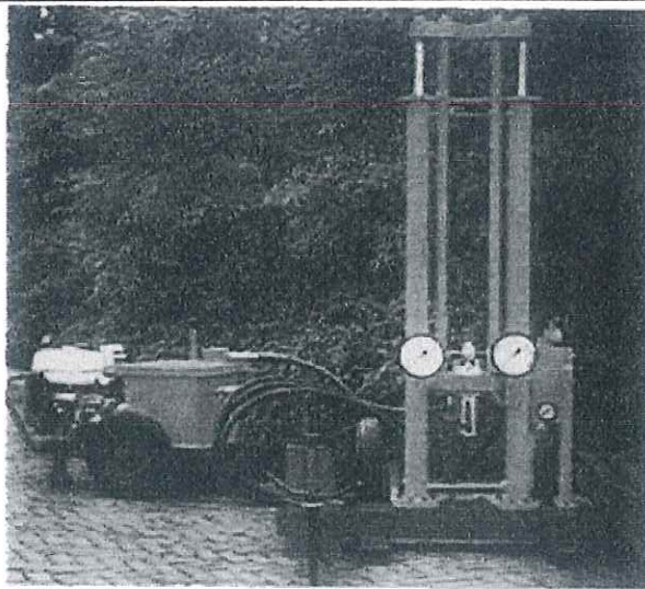
Thiết bị xuyên điện
