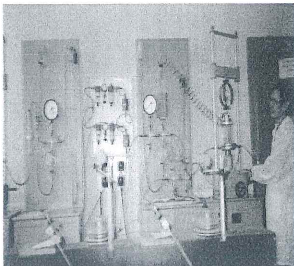
Thiết bị thí nghiệm nén 3 trục
